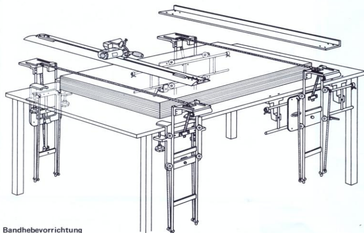
Bandhebevorrichtung
